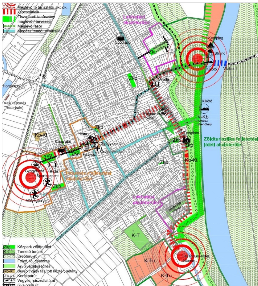
Zöldturisztikai javaslati tervlap – részlet
